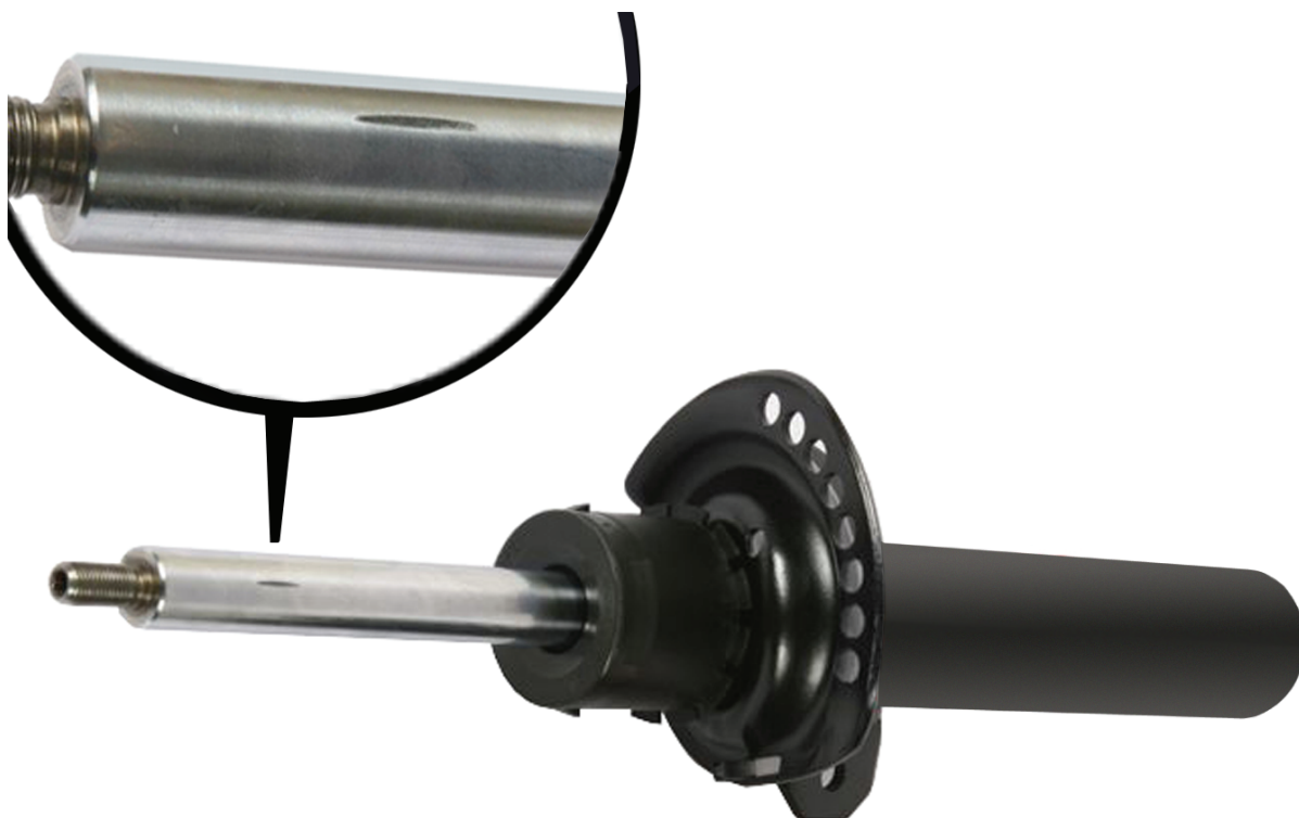
Rys. 1 Tłoczysko z rowkiem
