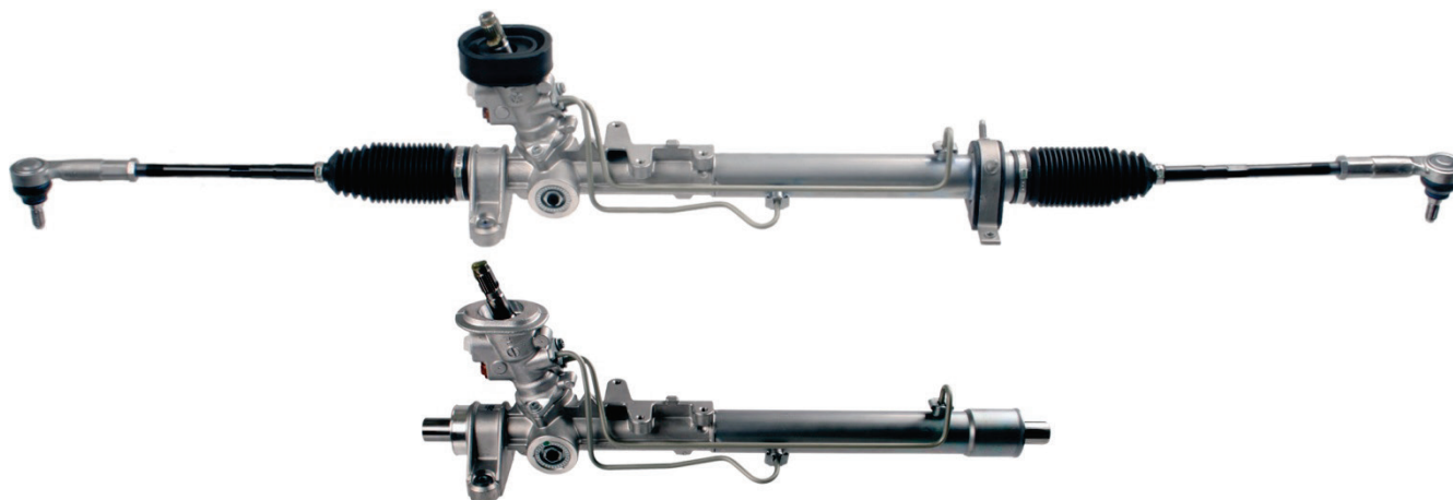
Rys. 1: Przekładnia kierownicza
